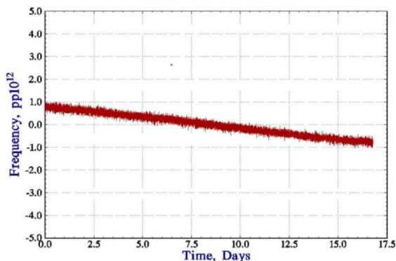
上图为16天连续运行的频率偏差曲线
